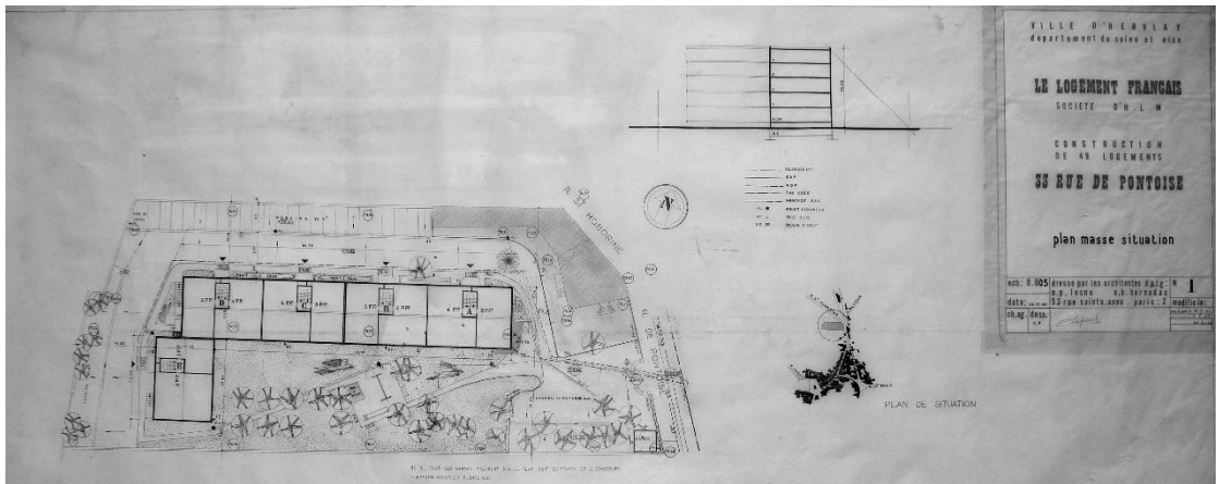
Plan de masse et de situation, calque. Fonds Lesné-Bernadac.
