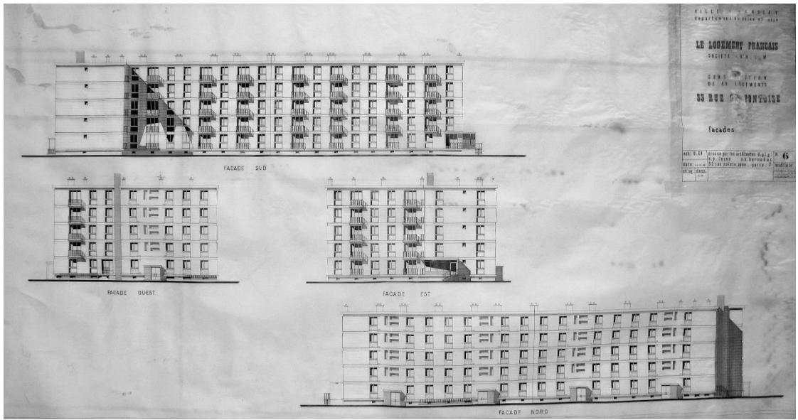
Façades, calque. Fonds Lesné-Bernadac.
