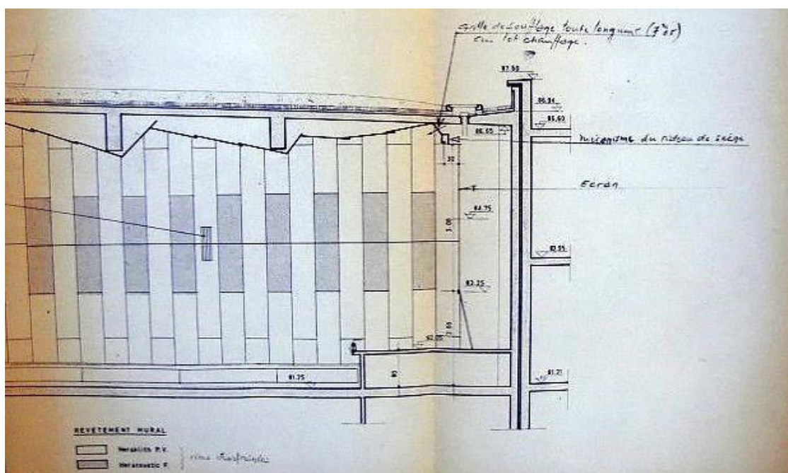
Plans en coupe de la salle et de la cabine de projection. Fonds Lesné-Bernadac.
