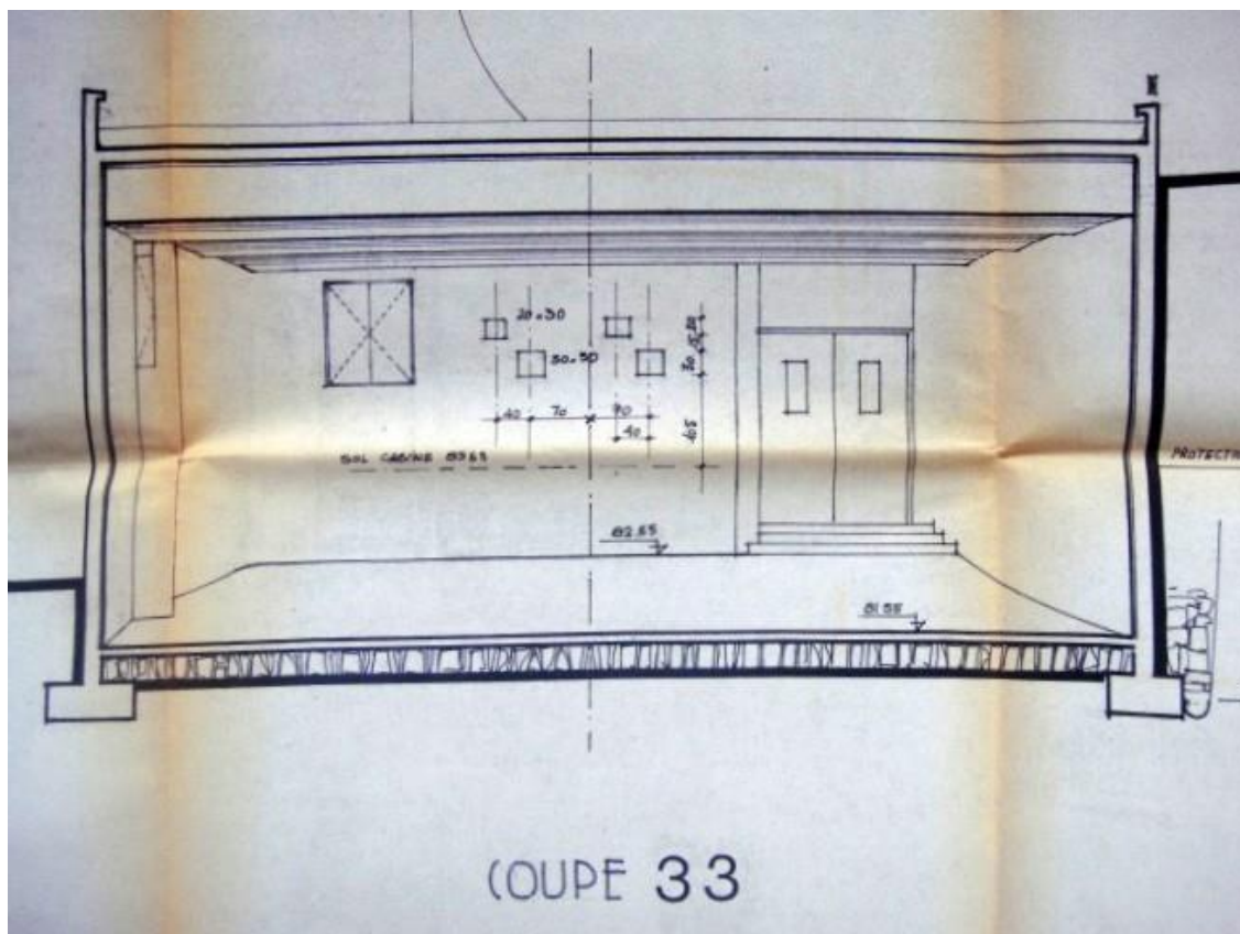
Plan en coupe de l'arrière de la salle et de la cabine de projection. Fonds Lesné-Bernadac.
