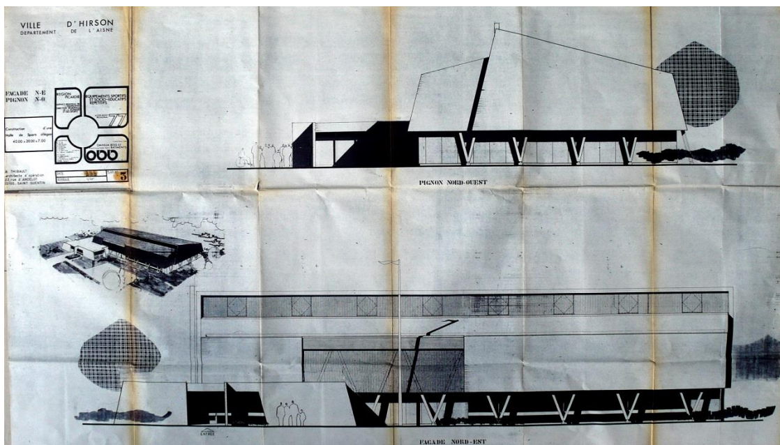
Façade principale et pignon. Fonds Lesné-Bernadac.
