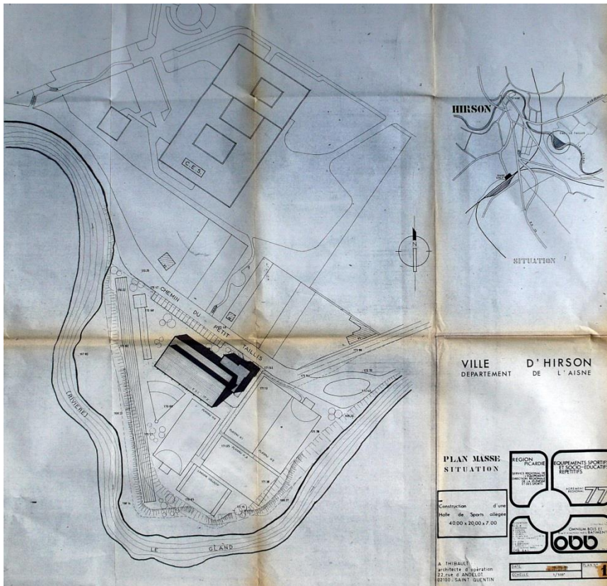
Plan de masse. Fonds Lesné-Bernadac.
