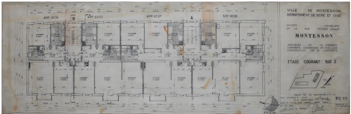
Plan d'étage courant, calque. Fonds Lesné-Bernadac.
